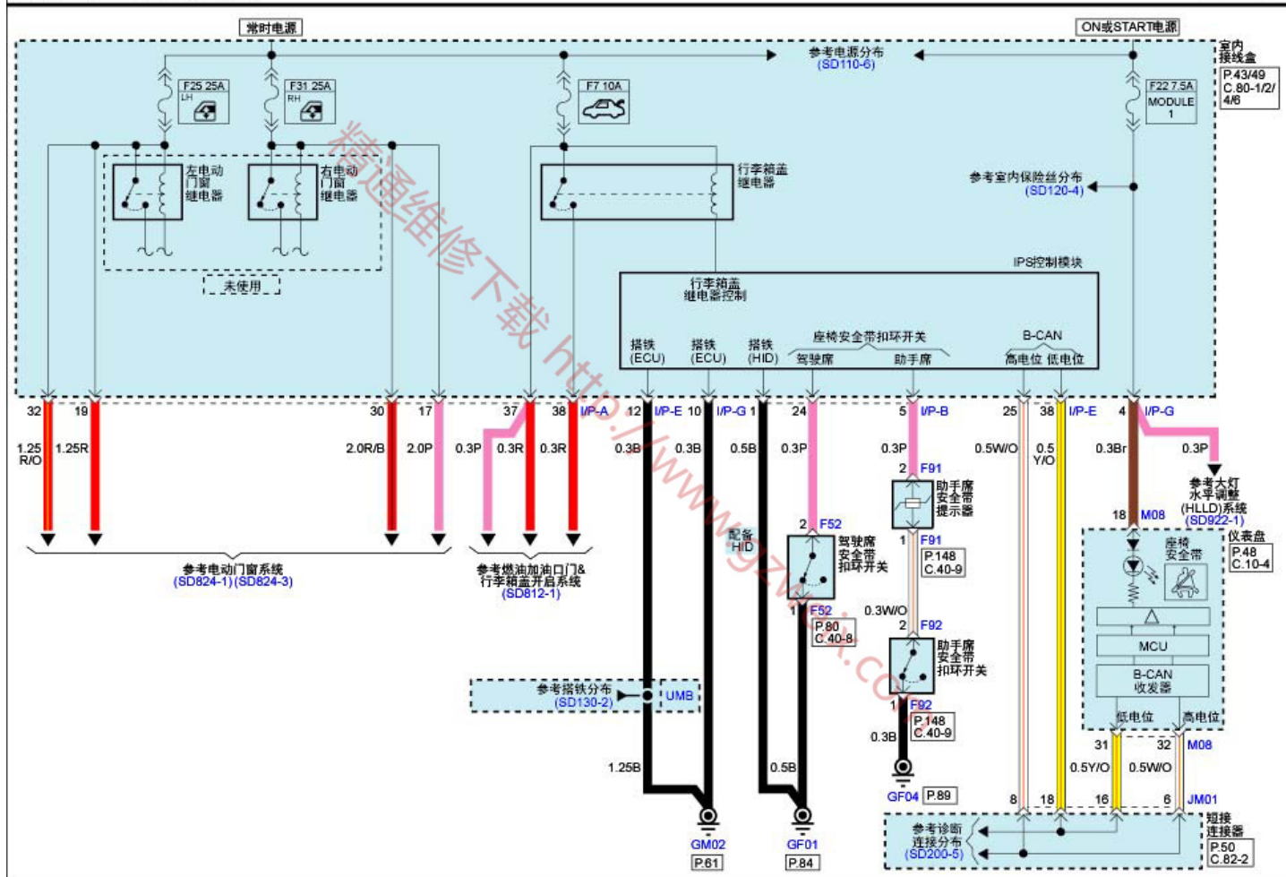
智能电源开关(IPS)系统(1)
